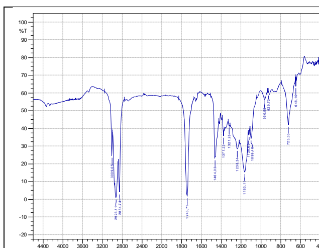
Рис.1. Спектр поглощения растительного масла.
