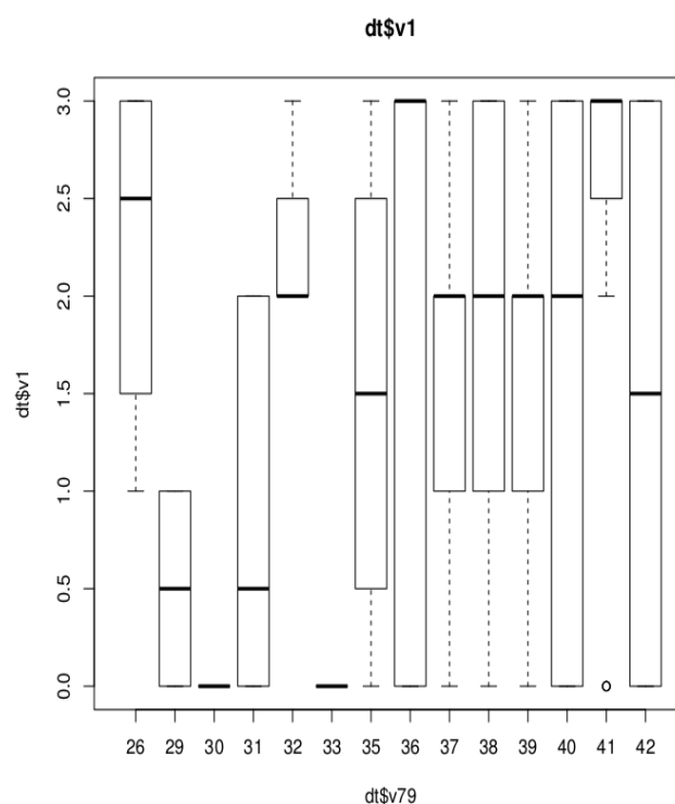
Рис. 1. Визуальный анализ межгрупповых различий течения гриппа у рожениц
