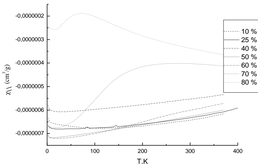
Рис.1. Температурные зависимости магнитной восприимчивости \chi_{\perp} кристаллов твердых растворов Sb_2Te_3 - Bi_2Te_3 . В рамке указано содержание Sb_2Te_3 в Bi_2Te_3-Sb_2Te_3 в мол. %.
